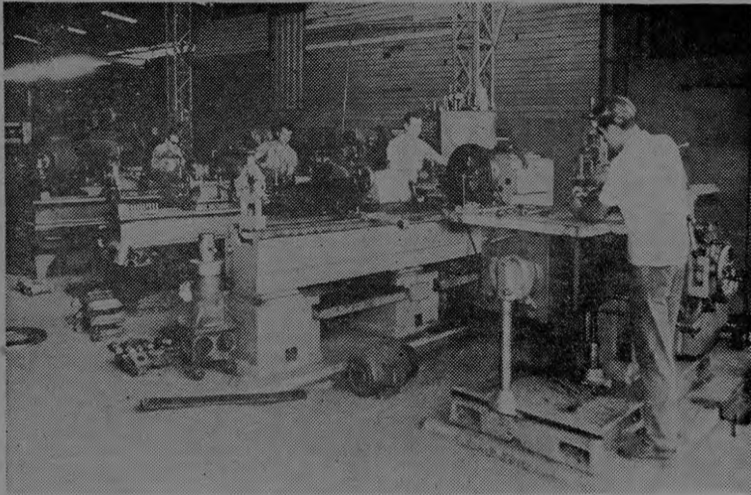
El taller Mecánico Industrial Chaves Ltda. de Grecia cuenta con moderna maquinaria, entre ellos 4 tornos, 2 taladros y 2 cepillos, cuya labor técnica realizan Freddy Quesada, Otto Ramirez, Franklin Arias y Orlando Arias.
