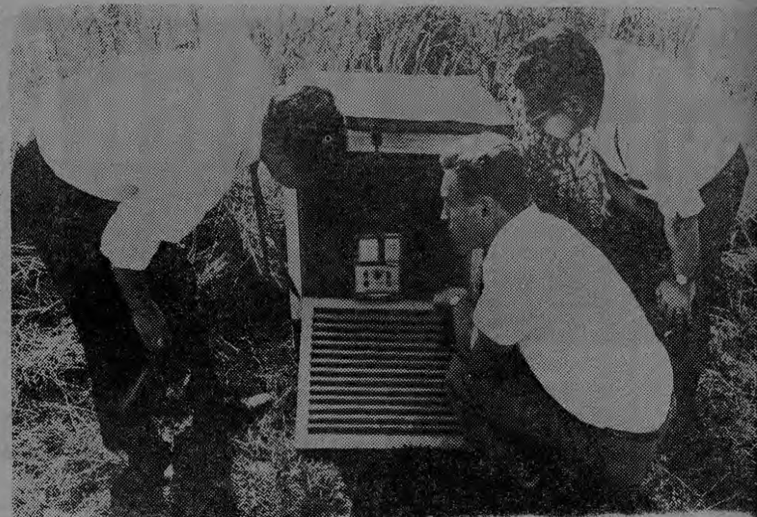
PARA ESTUDIAR el rendimiento de los estanques se instaló en el Instituto Experimental de Wielenbach un aparato que mide constantemente el contenido de oxígeno de los viveros, re-
